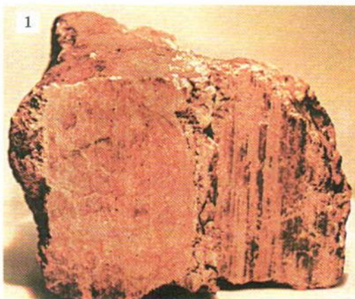
Рис. 238. 1 — метеорит с Марса; 2 — похожие на бактерии органические формы, обнаруженные в трещинах метеорита
