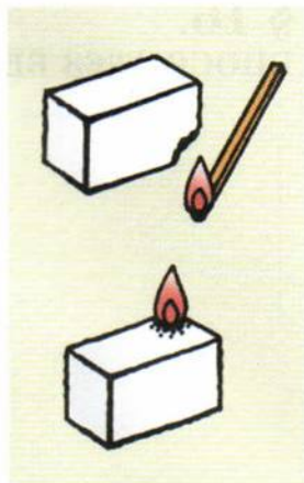
Рис 61. Горение сахара
