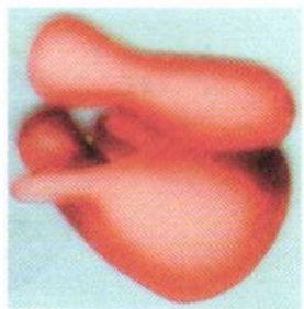
Рис. 50. Строение рибосомы
