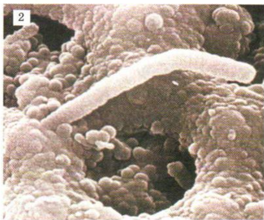
Рис. 238. 1 — метеорит с Марса; 2 — похожие на бактерии органические формы, обнаруженные в трещинах метеорита
