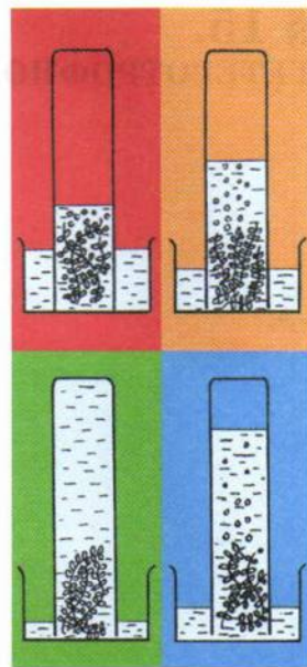
Рис. 58. Интенсивность фотосинтеза в разных спектрах света
